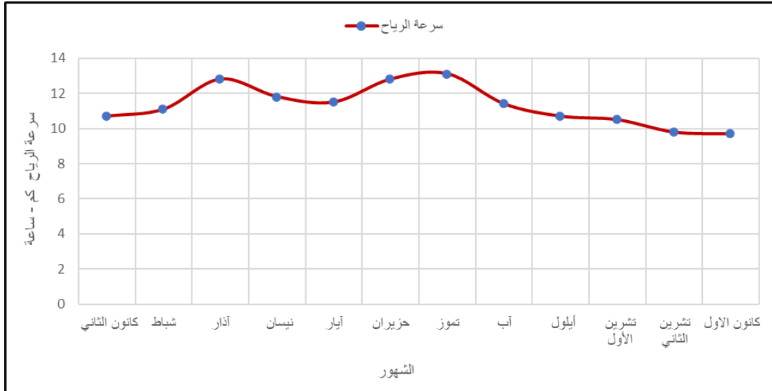
شكل (١١) معدلات سرعة الرياح في دولة الامارات العربية المتحدة لعام ٢٠٢١
