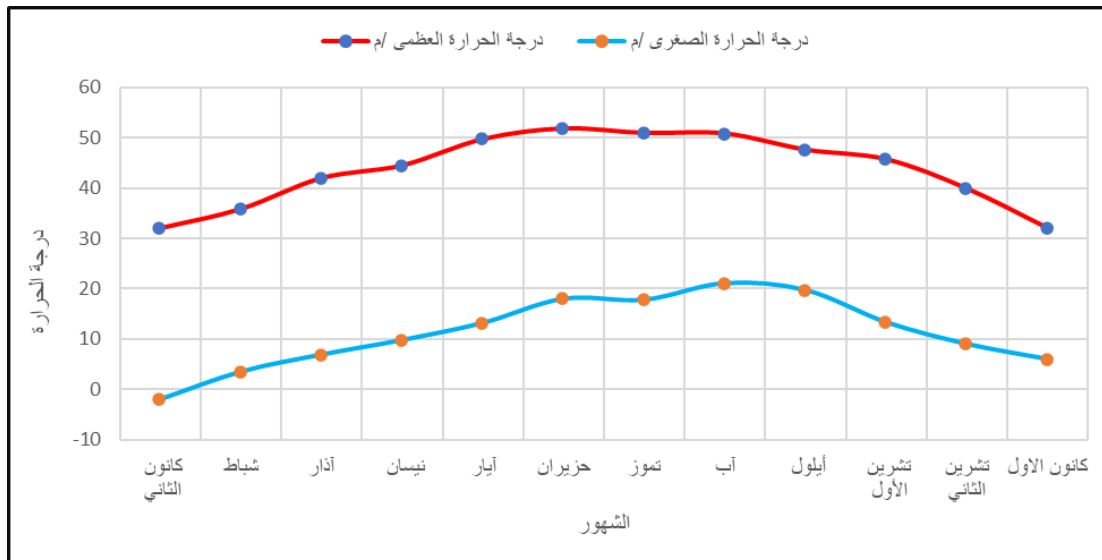
الشكل ( ٨ ) درجات الحرارة العظمى والصغرى خلال عام ٢٠٢١
