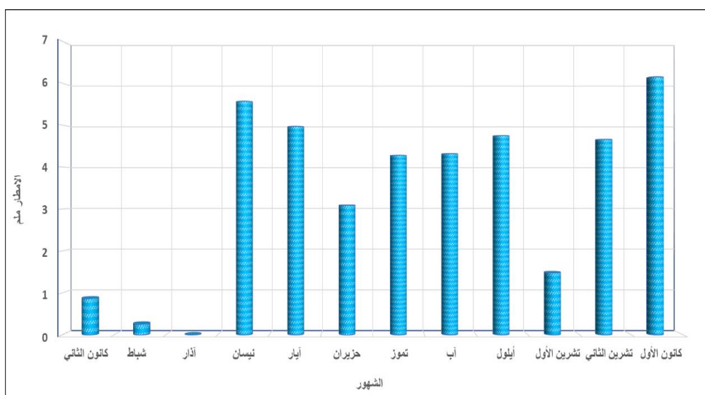
الشكل (١٠) معدلات الامطار لعام ٢٠٢١ في دولة الامارات العربية المتحدة
