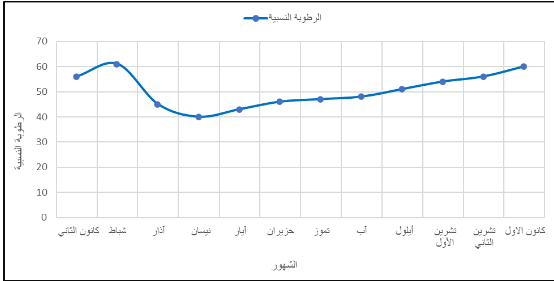
الشكل (٩) معدلات الرطوبة لعام ٢٠٢١
