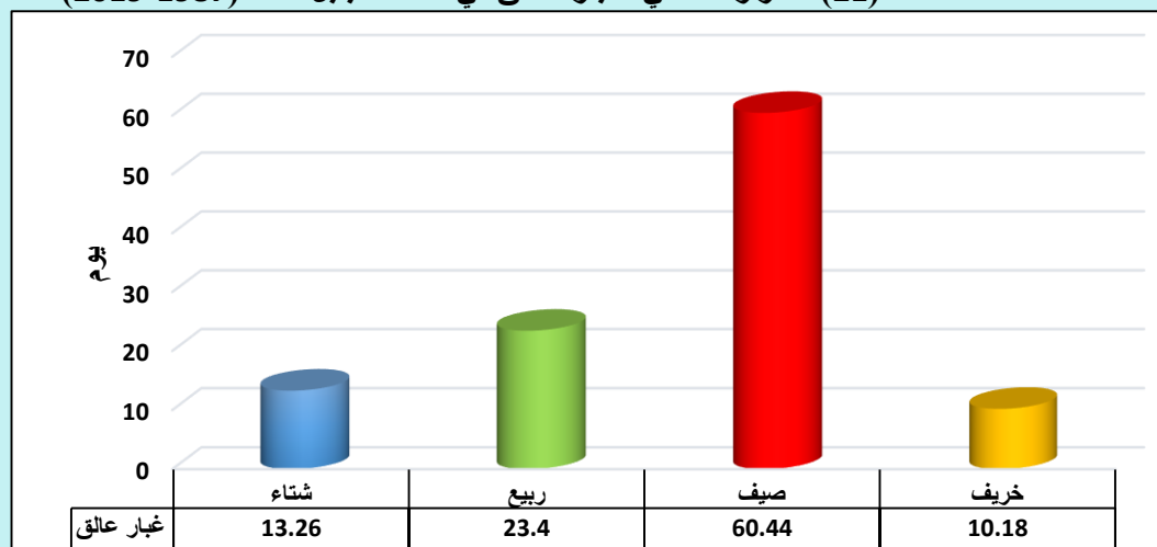
مخطط (21) التكرار الفصلي للغبار العالق في محافظة بابل للمدة (1987-2019)
