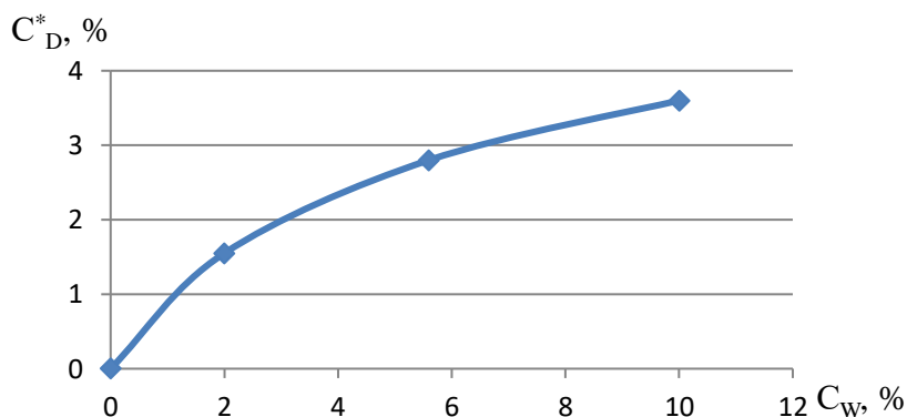
Рис. 2 - Равновесная зависимость концентраций извлекаемых веществ в экстрагенте и древесном сырье (шпоне)
