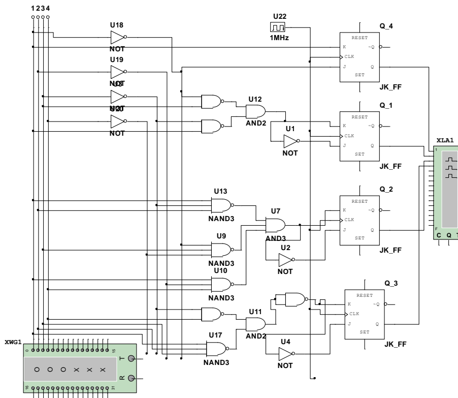
Рис. 1 – Схема счетчика-делителя в программе Multisim
