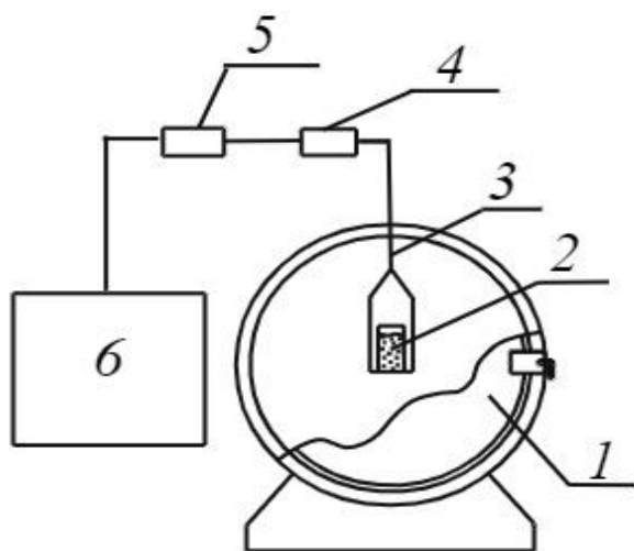
Рисунок 1 Схема установки удаления растворителя из суспензии наногрфита. 1 – сушильный шкаф, 2 – бюкс с суспензией наногрфита, 3 – подвес, 4 – тензодатчик, 5 – микроконтроллер, 6 - ПК
