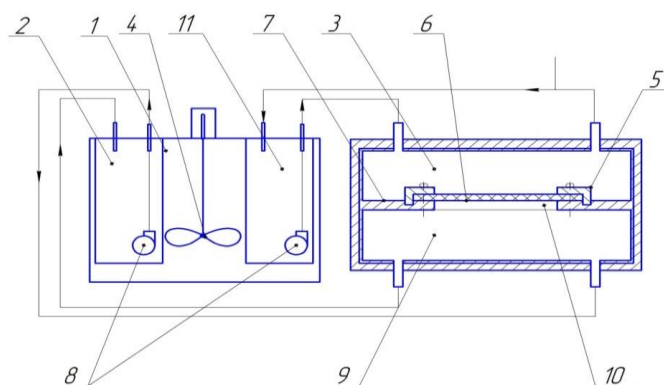
Рис. 1 Установка для определения коэффициента диффузии. 1 – термостат; 2, 11- буферные емкости; 3 – верхний отсек; 4 – мешалка; 5 – прижимной фланец; 6 – исследуемый образец; 7 – перегородка; 8 – центробежные насосы; 9 – нижний отсек; 10 – калиброванное отверстие
