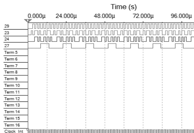
Рис. 2 – Временная диаграмма
